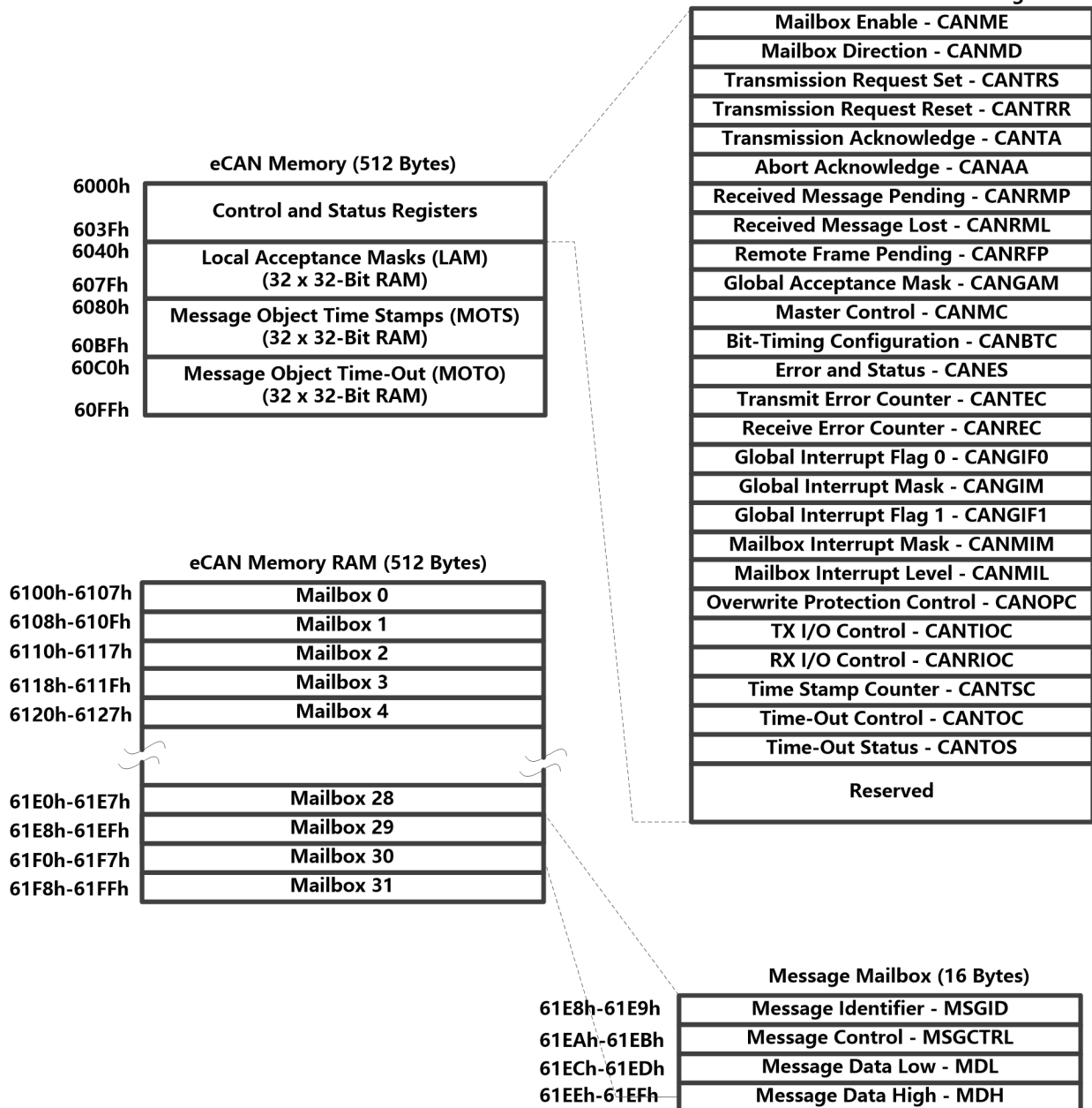
图图4-10 eCAN内存映射
