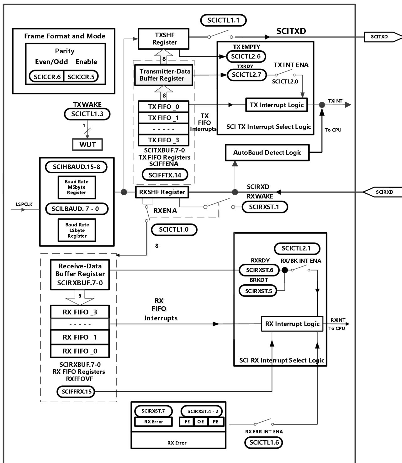
图4-7 SCI 模块框图
