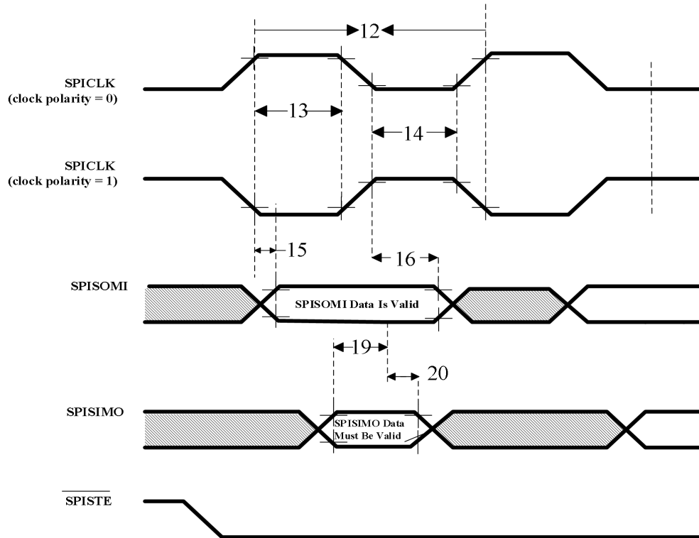
图6-25 SPI 从模式外部时序 (时钟相位= 0)
