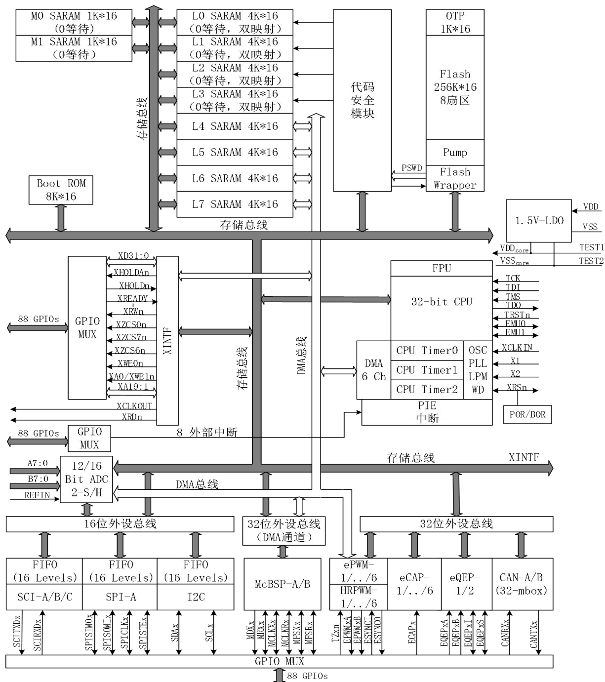
图 3-1 功能方框图
