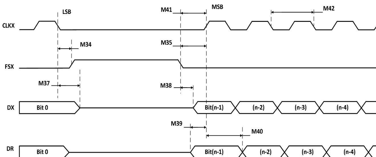
图 6-38 作为 SPI 主控或者受控时的 McBSP 时序: CLKSTP=11b, CLKXP=0
