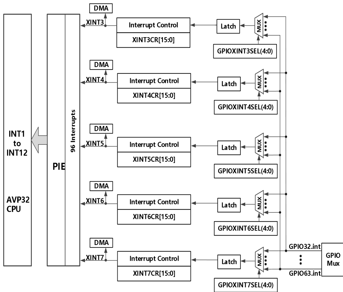
图 3-4 外部中断
