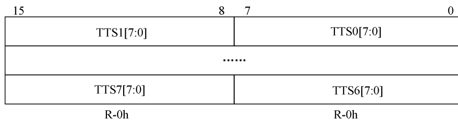
图 4-44 时间戳寄存器
