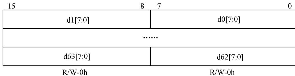
图 4-43 数据寄存器 0~3
