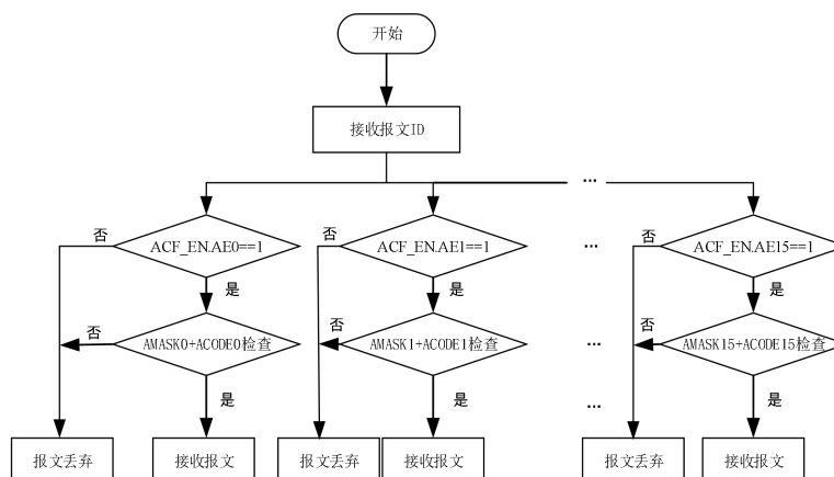
图 4-32 过滤流程图
