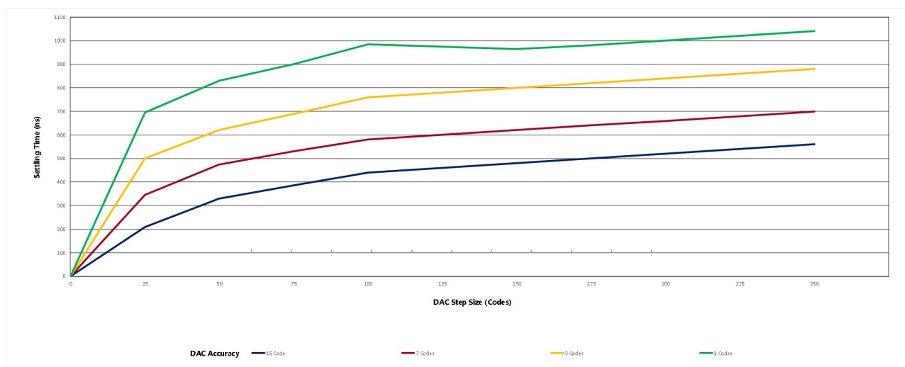
图4-13 DAC 稳定时间
