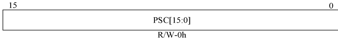
图 4-84 传输控制器预分频寄存器
