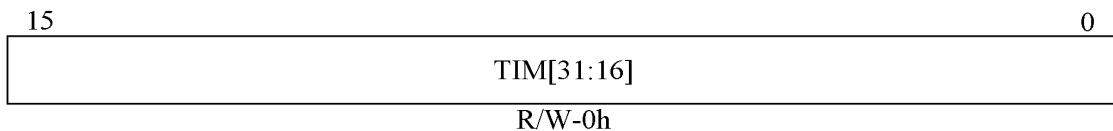
图 4-69 定时器计数器 1 寄存器
