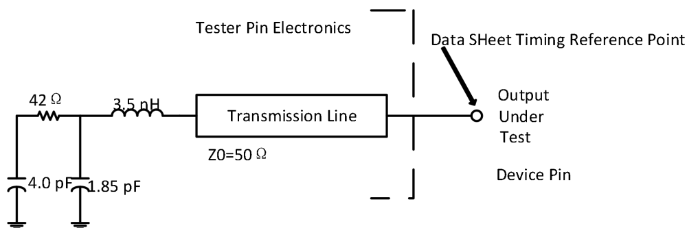
图 5-5 3.3V 测试负载电路
