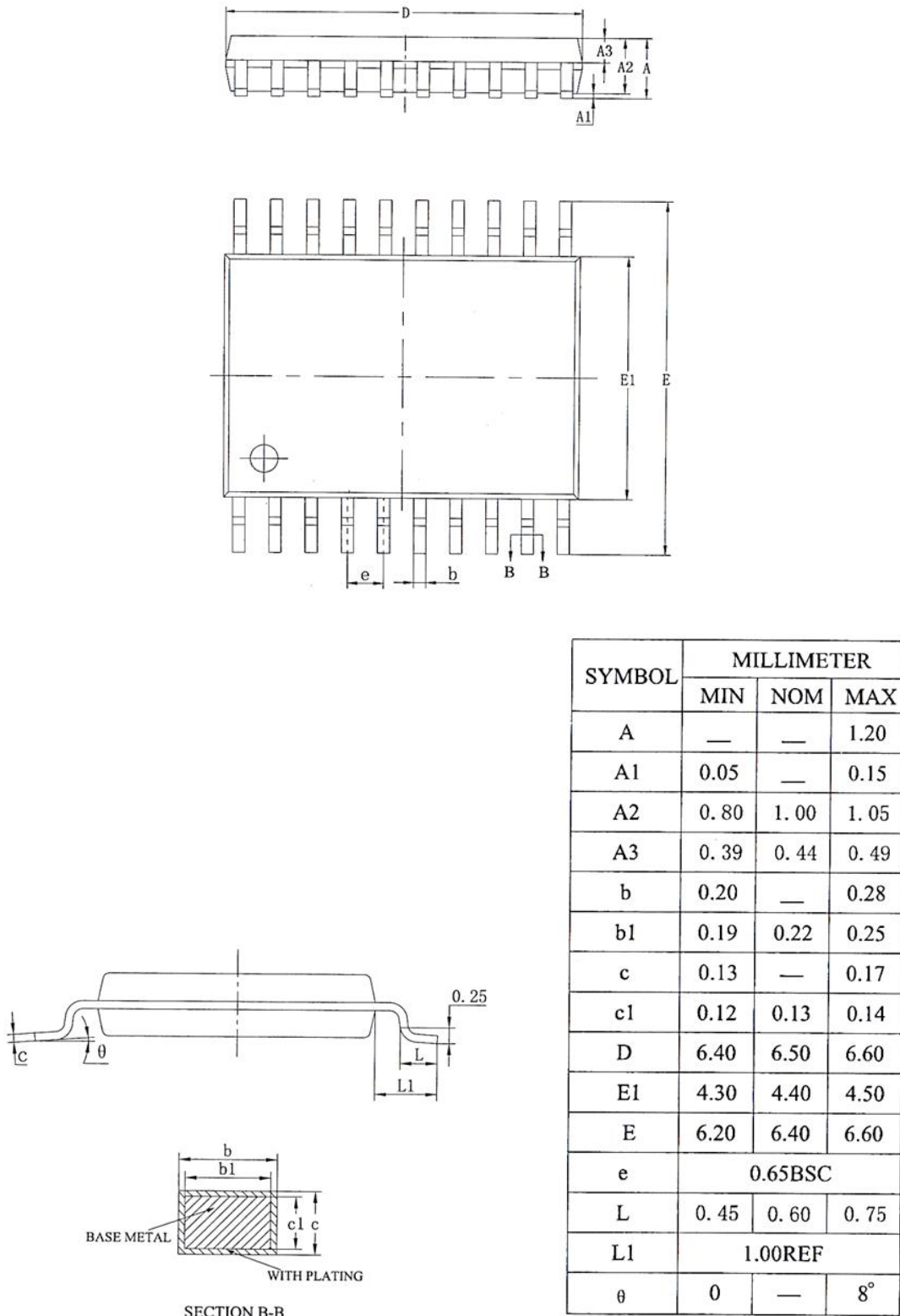
图 6-6 TSSOP20 封装外形尺寸图
