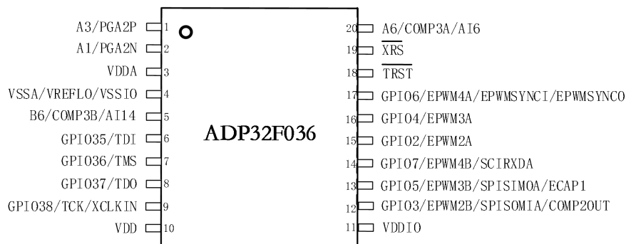
图 2-7 ADP32F036 芯片 TSSOP20 封装引脚排布
