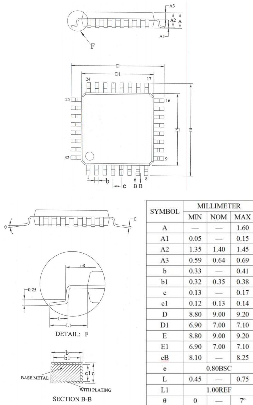
图 6-4 LQFP32 封装外形尺寸图
