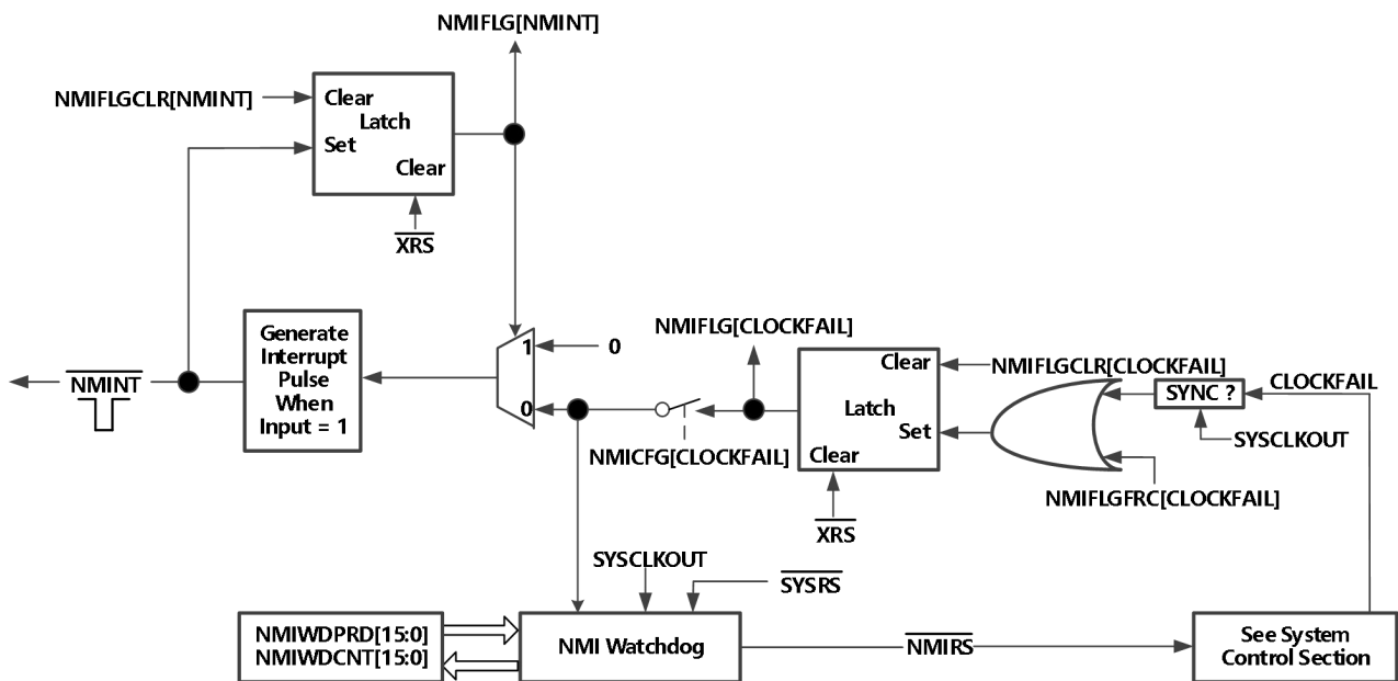
图 3-11 NMI - 看门狗
