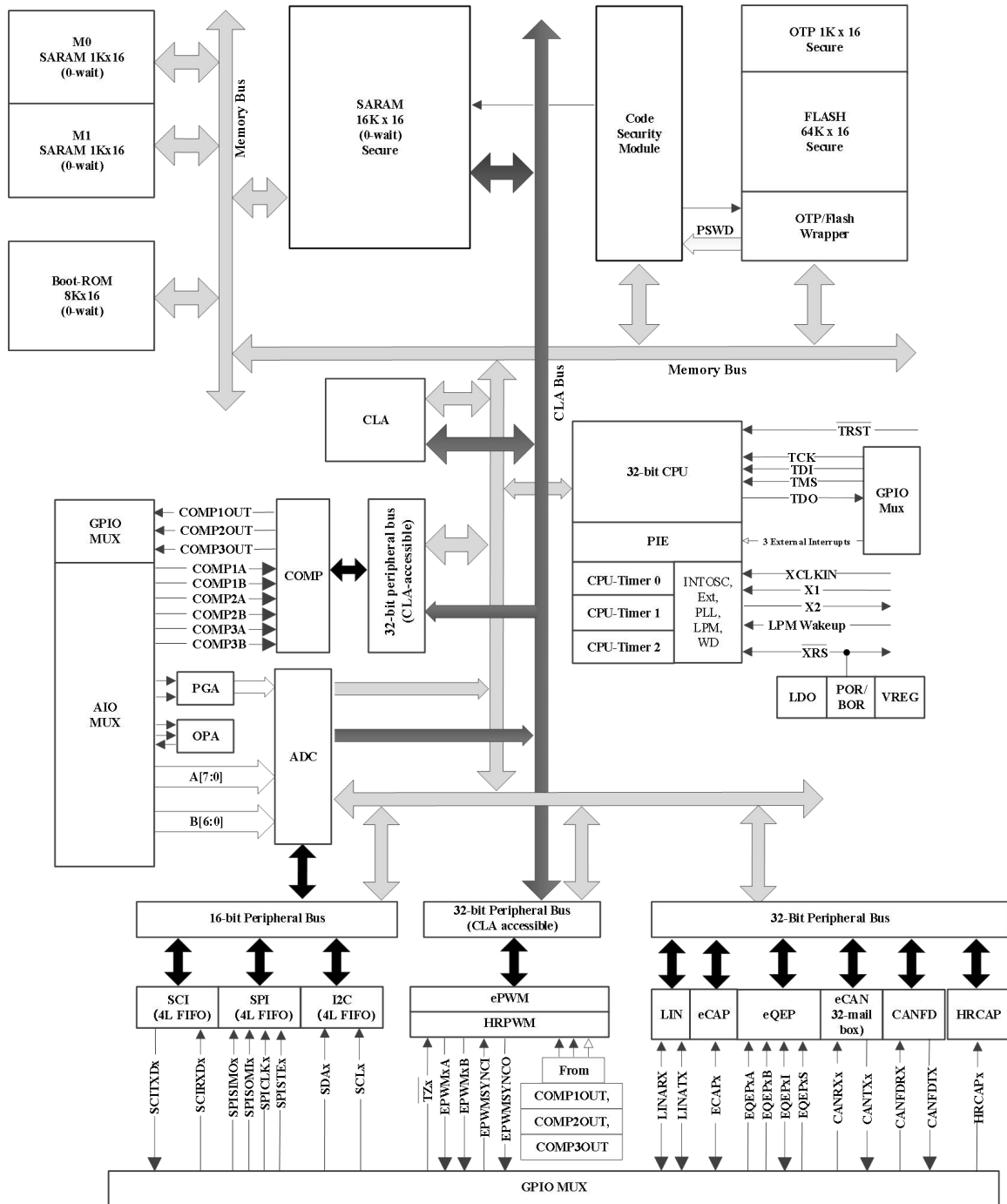
图 3-1 功能框图
