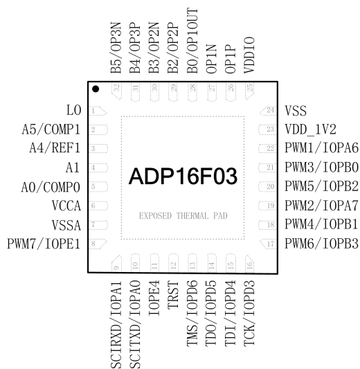
图 3-4 QFN32 封装引脚排布
