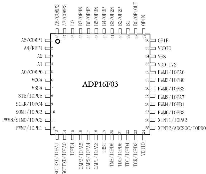
图 3-1 LQFP48 封装引脚排布
