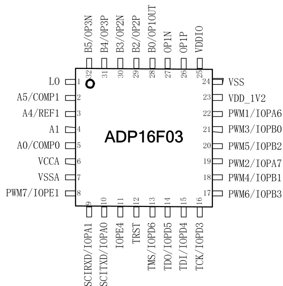
图 3-3 LQFP32 封装引脚排布
