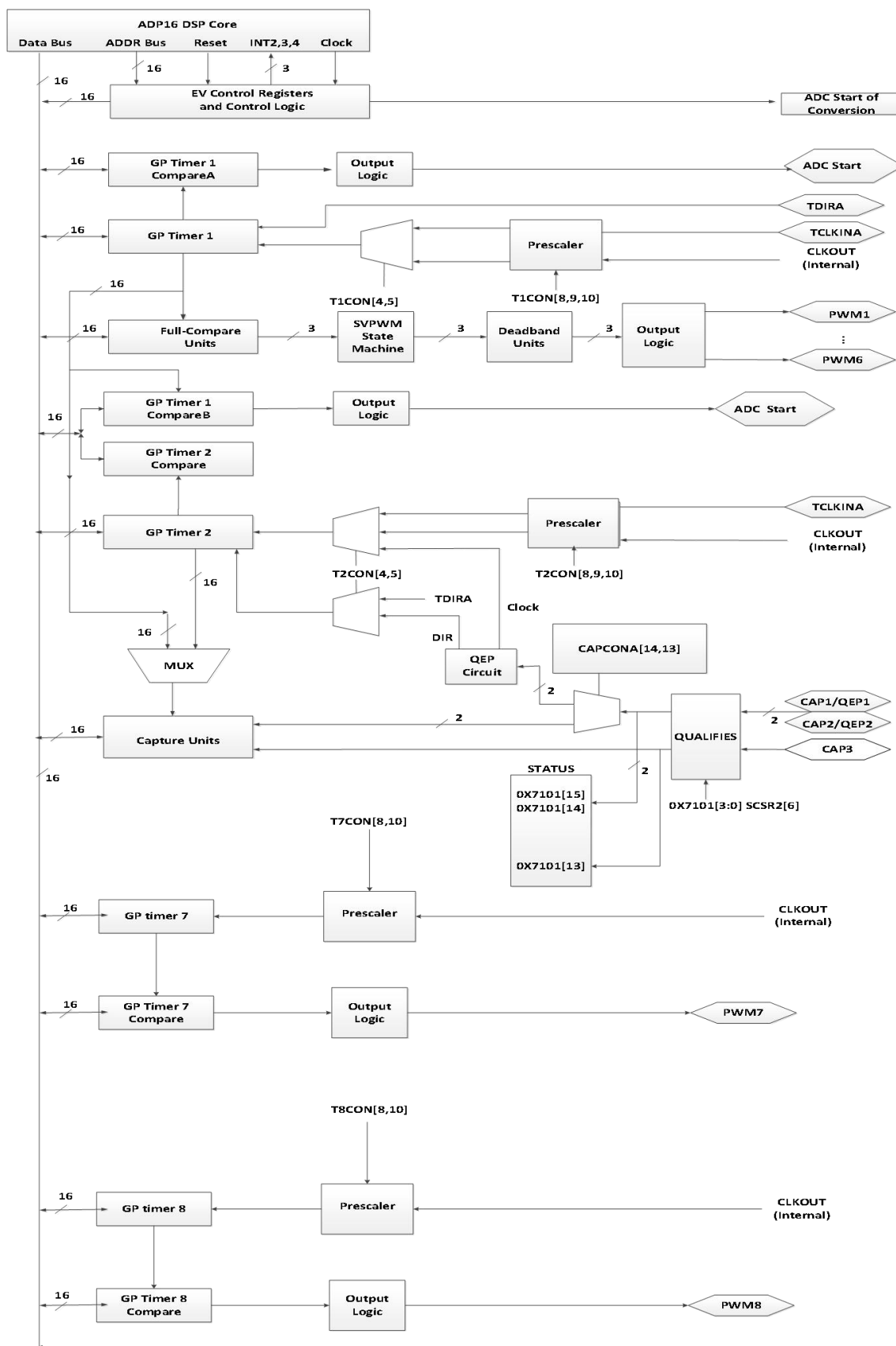
图 14-1 事件管理器模块 (EM1) 结构框图
