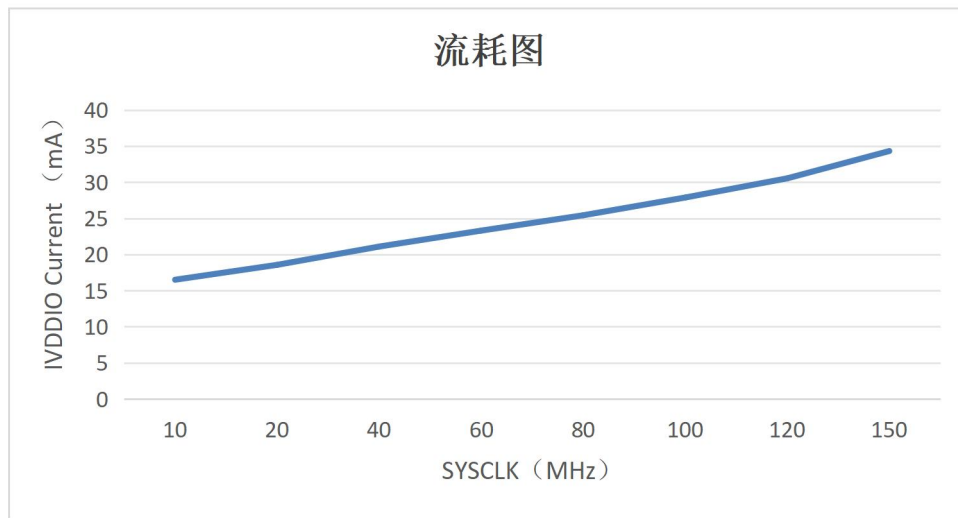
图 20-1 ADP16F03 在频率范围内的典型电流消耗（使能外设时钟）
