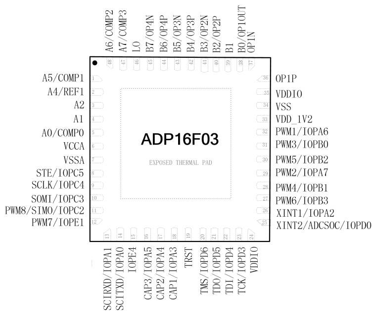
图 3-2 QFN48 封装引脚排布
