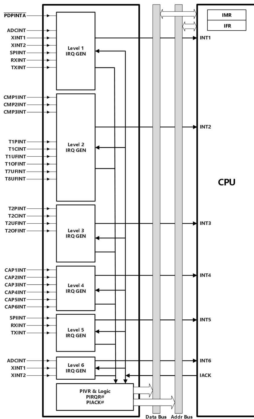
图 8-1 硬件中断 PIE 结构框图
