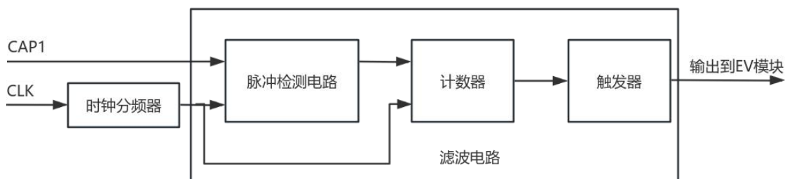
图 18-1 CAP1 数字延时滤波示意图
