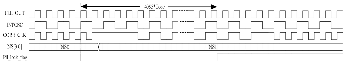
图 7-2 PLL 时钟 bypass 控制部分信号时序图
