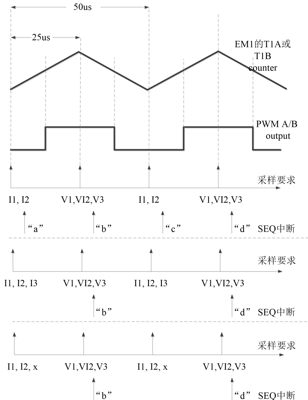
图 15-3-6 定序转换期间的中断操作
