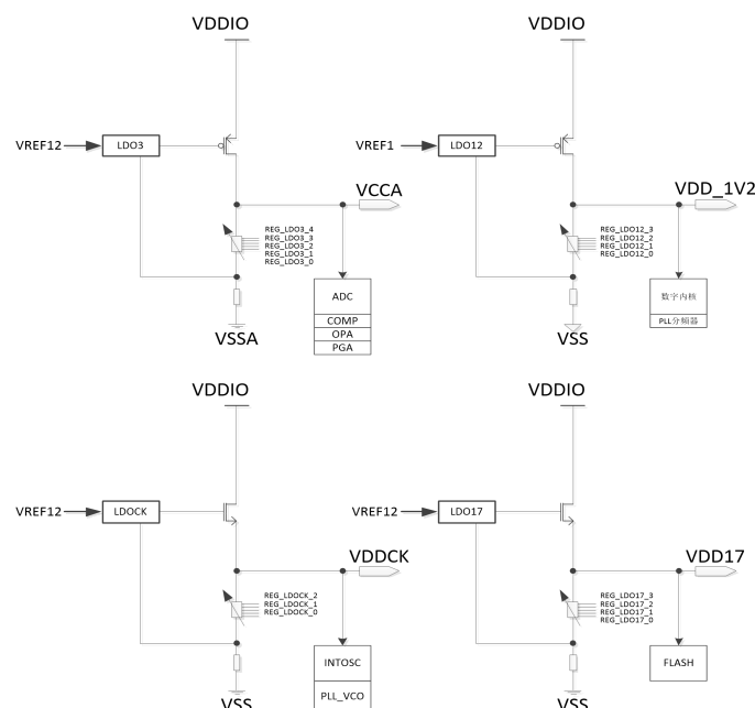
图 19-1-1 芯片各模块供电框图
