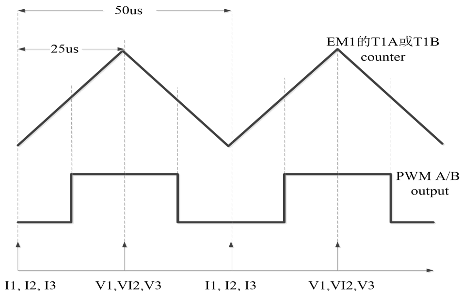
图 15-3-5 EM1_T1A/EM1_T1B 触发启动排序器的示例
