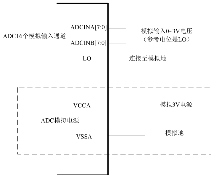
图 15-2-2 ADC 电源的引脚连线
