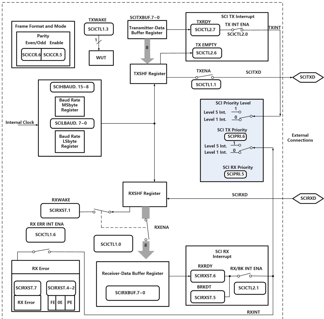
图 12-1 SCI 模块结构框图
