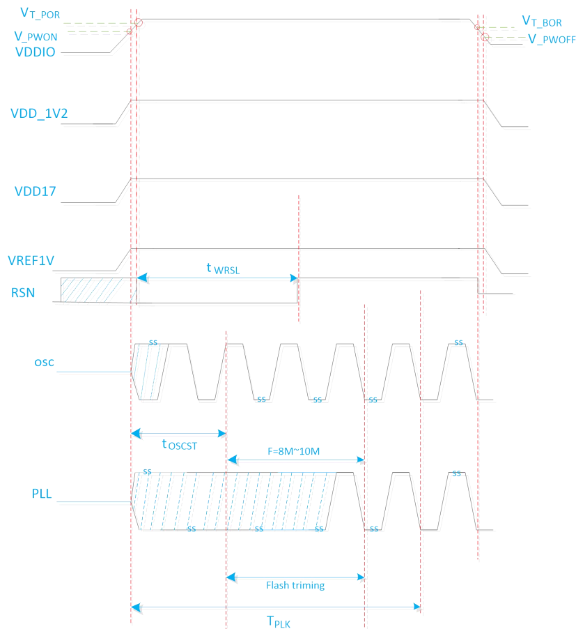
图 19-1-2 BORPOR 上电下电复位时序图
