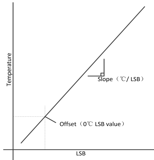
图 15-6-1 温度传感器传递函数
