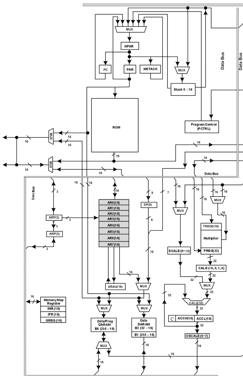
图 5-1 CPU 功能模块框图
